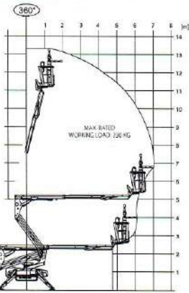
JLG X13J PLUS
