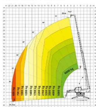
LASTDIAGRAM BIJ UITGESCHOVEN STEMPELS 360°
