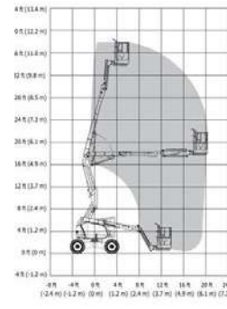
DIESEL 340AJ
