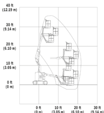
ELECTRISCH JLG 300AJP
